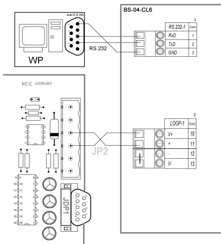
Подключение ГНК EUROPUMP по интерфейсу 2-WIRE.
