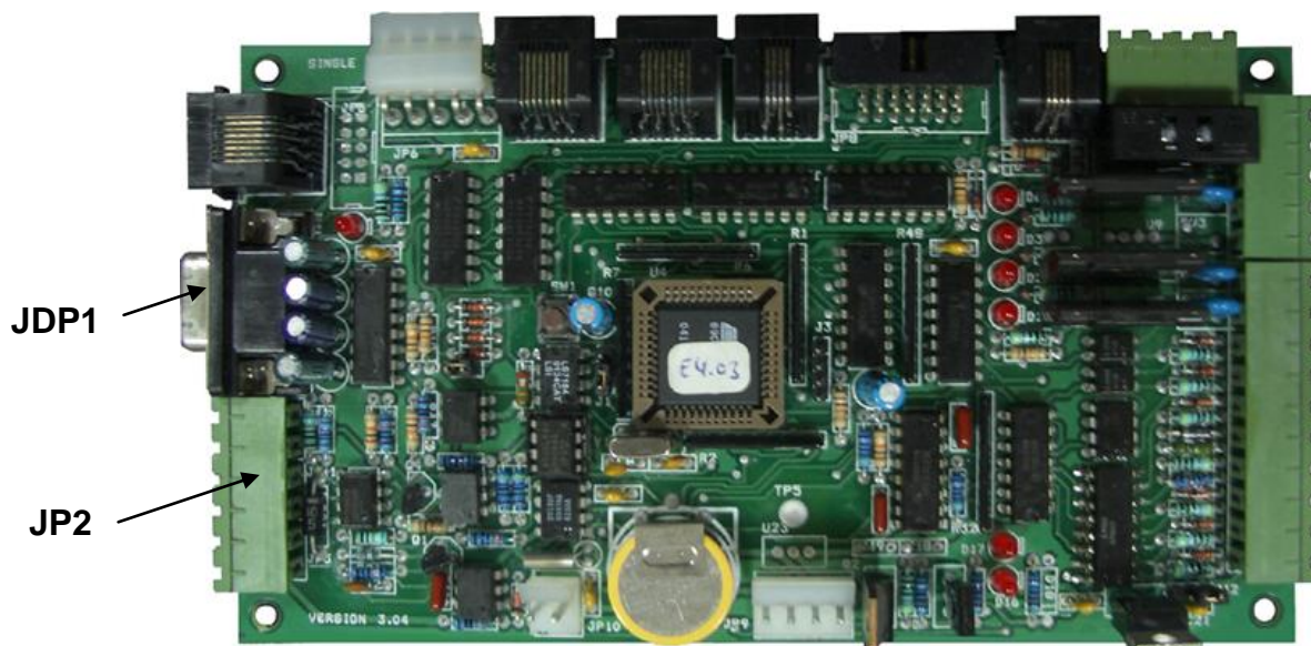
Подключение ГНК EUROPUMP по интерфейсу 2-WIRE.
